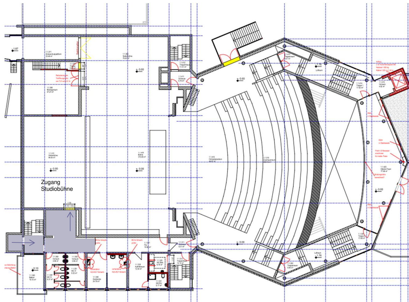
Grundriss Bühnengeschoss
