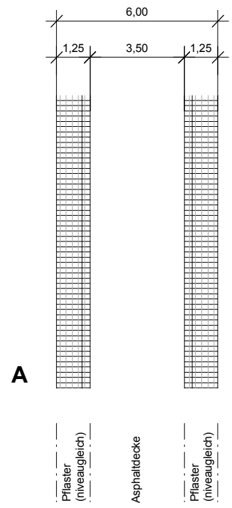
Planstrasse M. 1: 200
